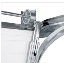
Entrebâillement du panneau supérieur (en option)
