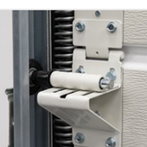
Charnières blanches assurent un aspect uniforme de l'intérieur de votre porte
