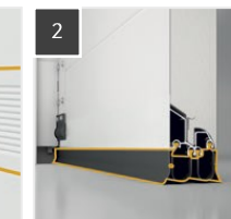
2 Joint d'étanchéité inférieur à double lèvres
