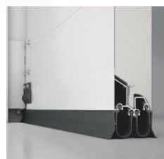
Joint inférieur à double lèvres
