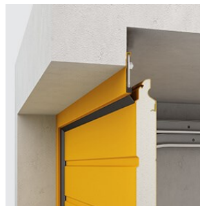
Installation derrière la baie - cache rénovation (2.0)
