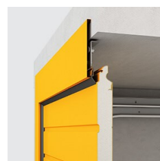
Installation dans la baie – cache devant la baie
